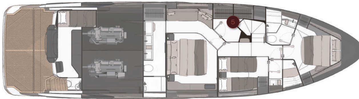
CONFIGURAÇÃO DE TRÊS CABINES Configuration three cabin
