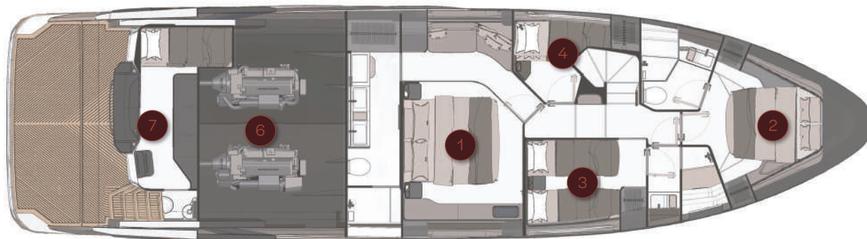
CONFIGURAÇÃO DE QUATRO CABINES Configuration four cabin
